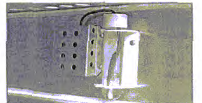
Sensor tipo NTC (Simula a temperatura da vacina no momento)
